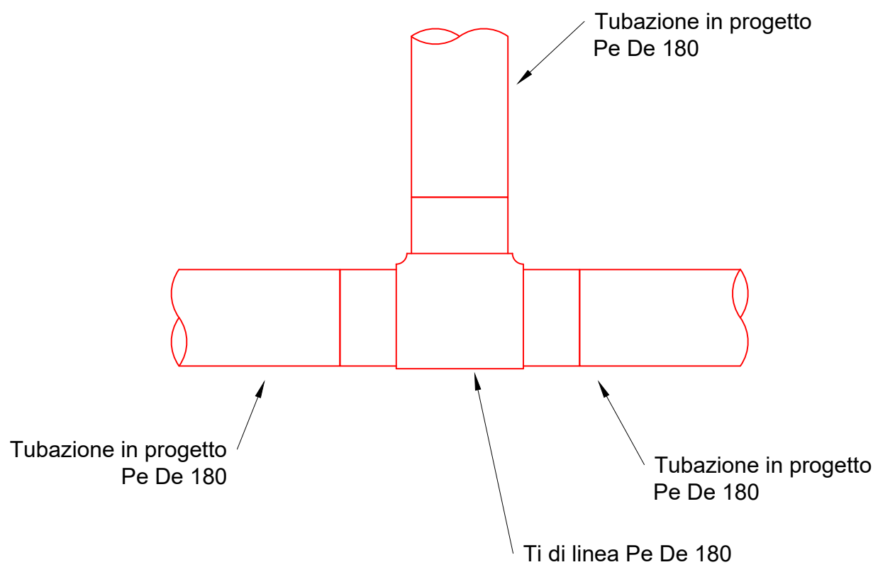
Tipologico 3 Collegamento a Ti di linea Pe De 180 Nodi 5-26-27-35-38-46-48
