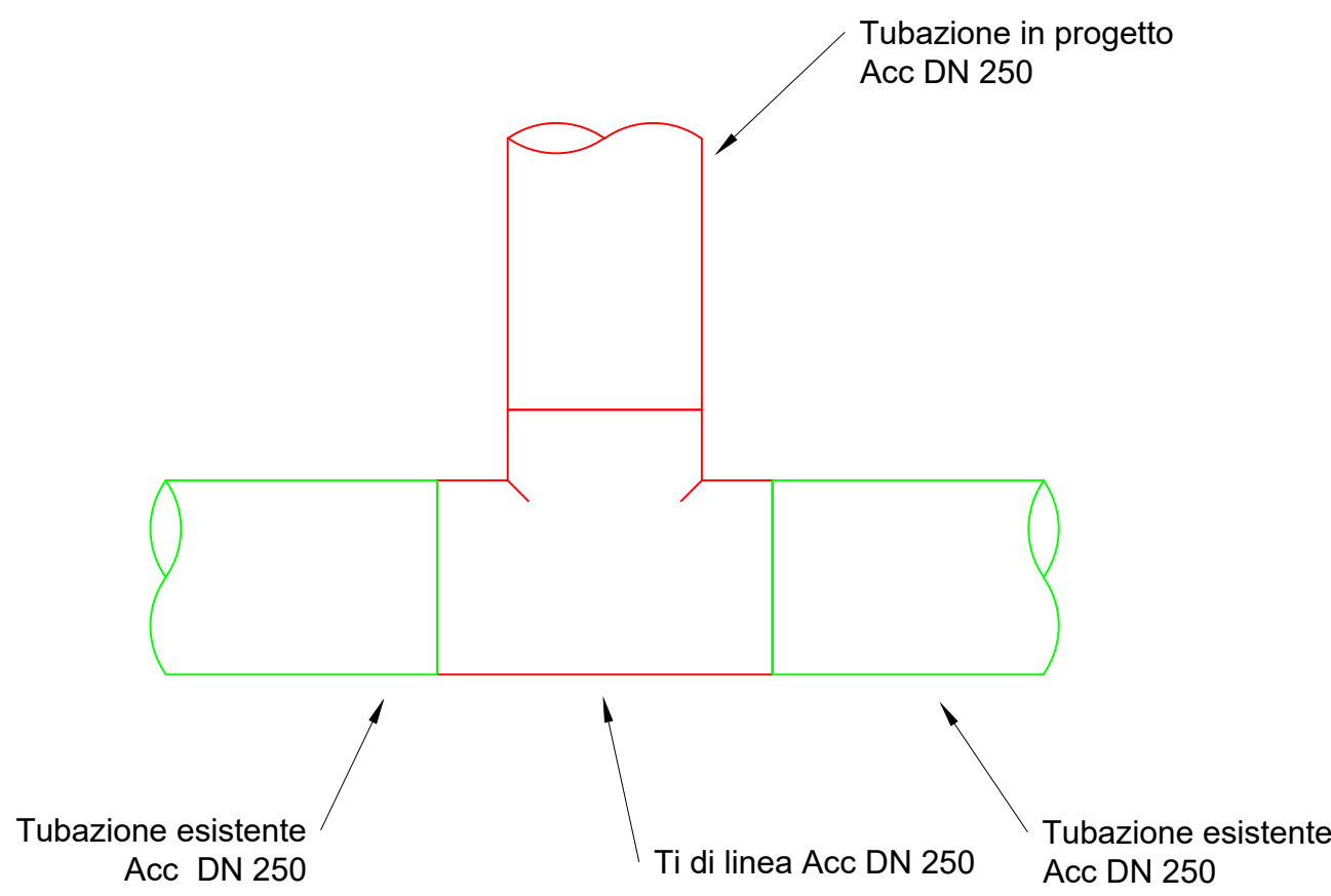
Tipologico 9 Collegamento a Ti di linea Acc DN 250 Nodo 13
