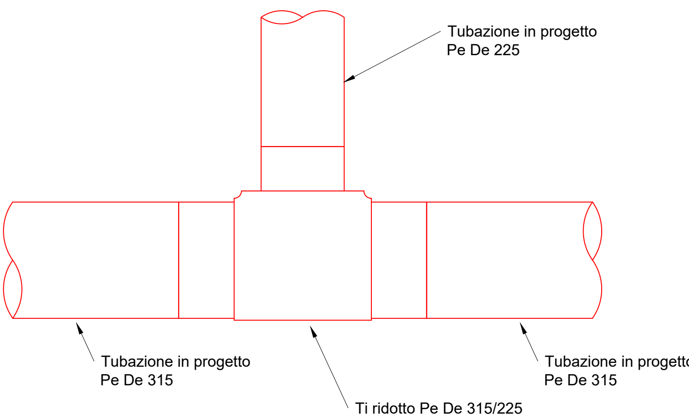
Tipologico 8 Collegamento a Ti ridotto Pe De 315/225 Nodi 11-12-14-15-16-19-25 32-41-64-67-73-74-75-76-77 78-79-88-89-90-91-92-93-94-95
