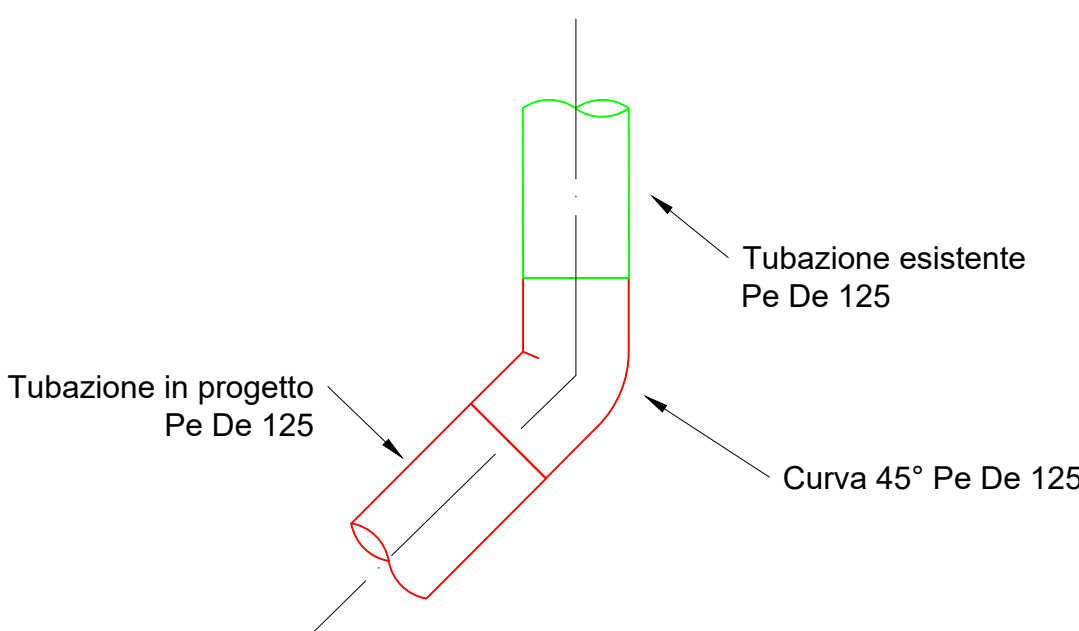
Tipologico 16 Collegamento in linea curva 45° Pe De 125 Nodi 69-72
