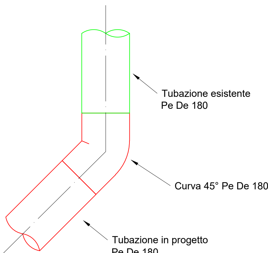
Tipologico 10 Collegamento in linea curva 45° Pe De 180 Nodi 18-31
