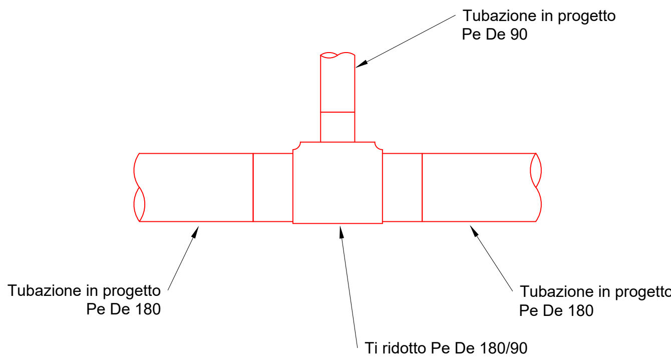
Tipologico 2 Collegamento a Ti ridotto Pe De 180/90 Nodi 2-3-4-17-29-30-33-34-36-37-39-42-43-44-45 49-50-51-52-53-55-56-60-61-62-63-80-81-82-83-84-85-86
