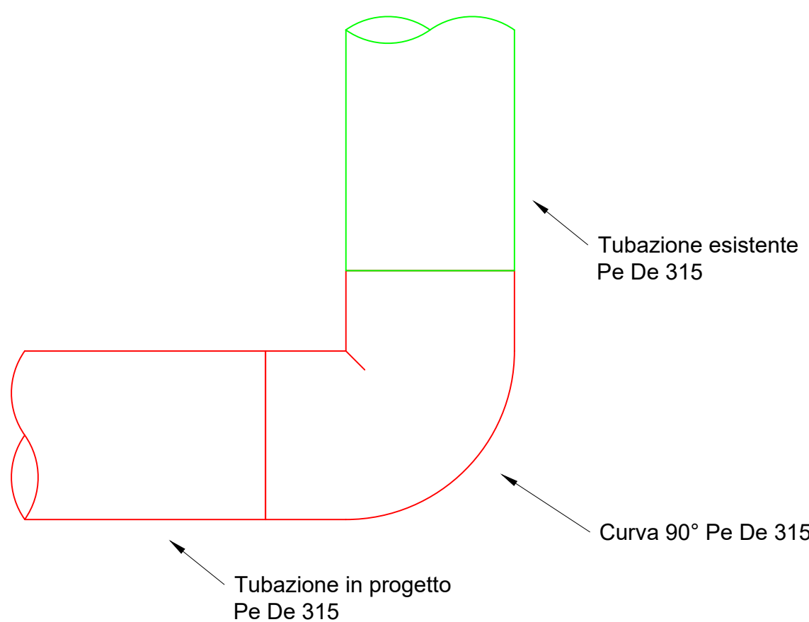
Tipologico 14 Collegamento in linea curva 90° Pe De 315 Nodo 66
